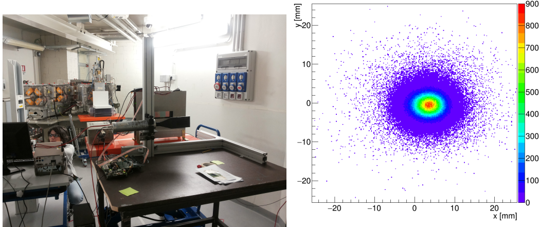
Fig. 6.8.2. Il fascio di protoni da 220 MeV osservato con un tracciatore al silicio seguita da un calorimetro – apparato utilizzato da Carlo Civinini, INFN Firenze.
